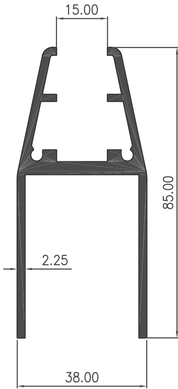
Section No : 6103
