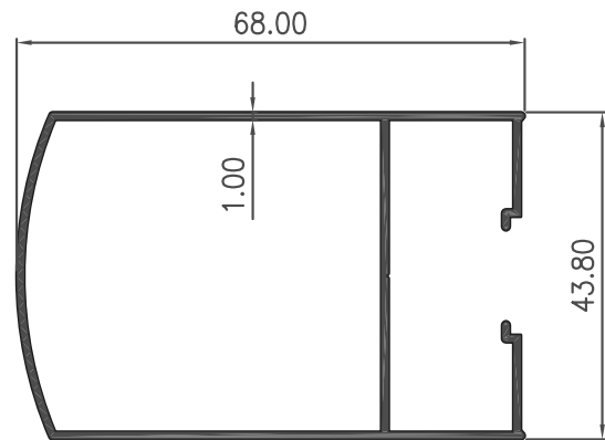
Section No : 2008
