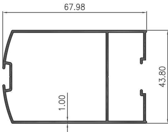
Section No : 2007
