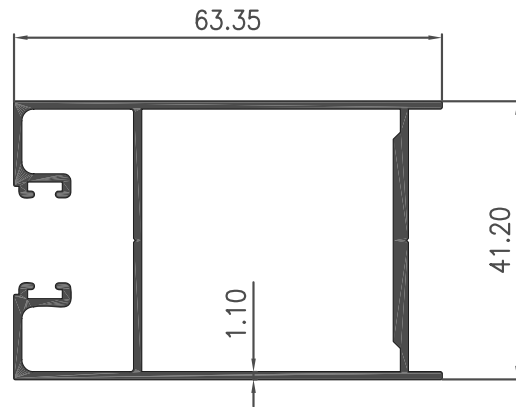
Section No : 2011
