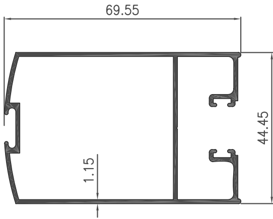
Section No : 2001
