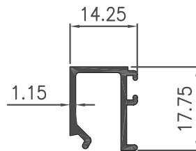
Section No : 2003
