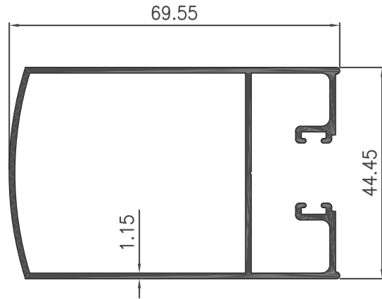
Section No : 2002
